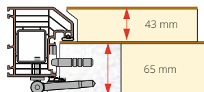
Schemat zespolenia ościeżnicy ze skrzydłem 3D
